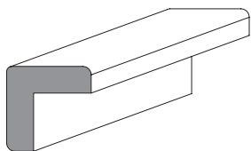
T4-201 1 x 1
